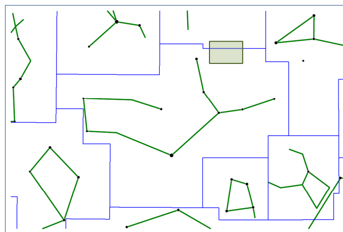
Vir – Cluster
