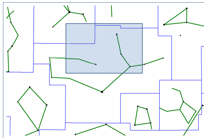
Vir 1-2
