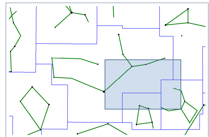
Vir 2-3
