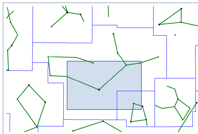
Vir 2-2
