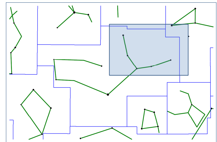
Vir 1-3
